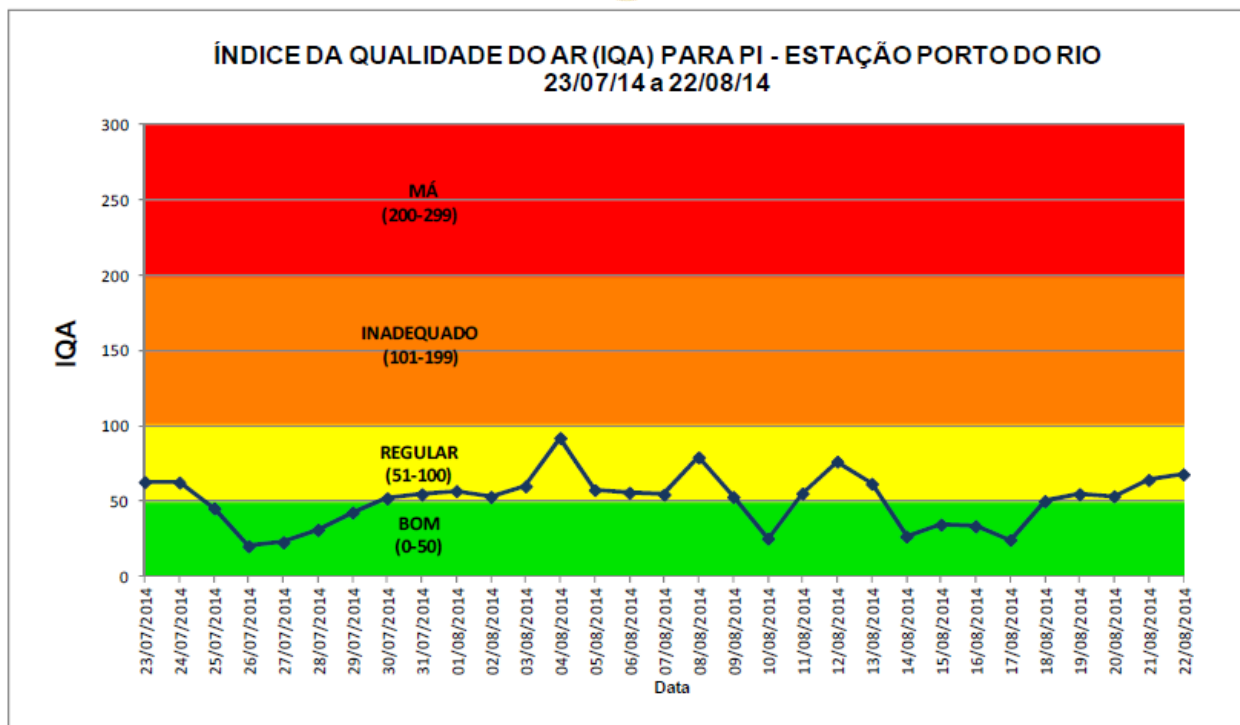
Figura: Variação temporal dos Índices de Qualidade do Ar para Partículas Inaláveis no período de 23/07/14 a 22/08/14 (Fonte: JCTM). Pontos de Medição: Praça Mauá e Inca.
