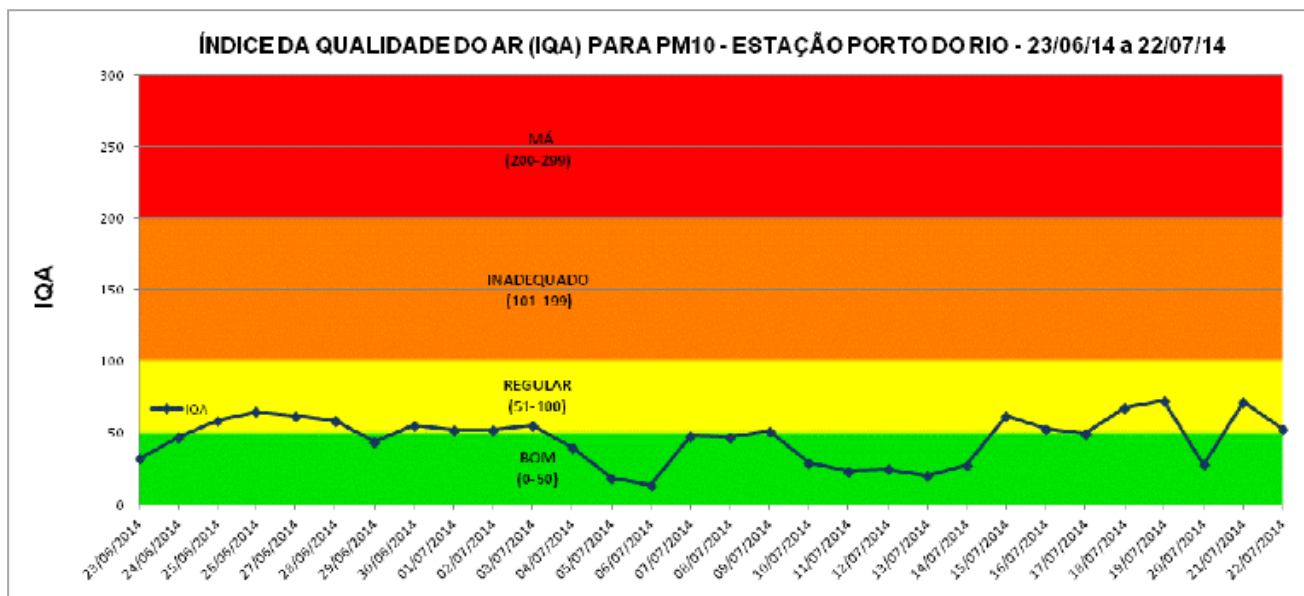
Figura: Variação temporal dos Índices de Qualidade do Ar para Partículas Inaláveis no período de 23/06/14 a 22/07/14 (Fonte: JCTM). Ponto de Medição: Praça Mauá.
