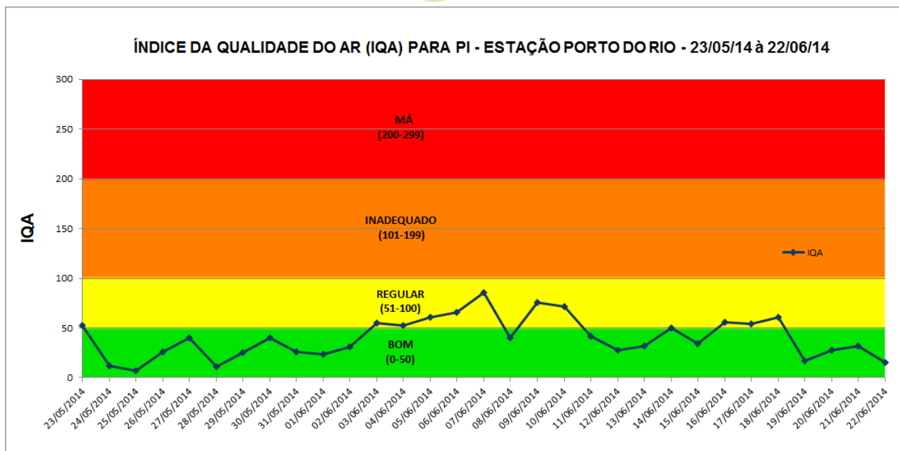
Figura 1: Variação temporal dos Índices de Qualidade do Ar para Partículas Inaláveis no período de 23/05/14 a 22/06/14 (Fonte: JCTM). Ponto de Medição: Praça Mauá.
