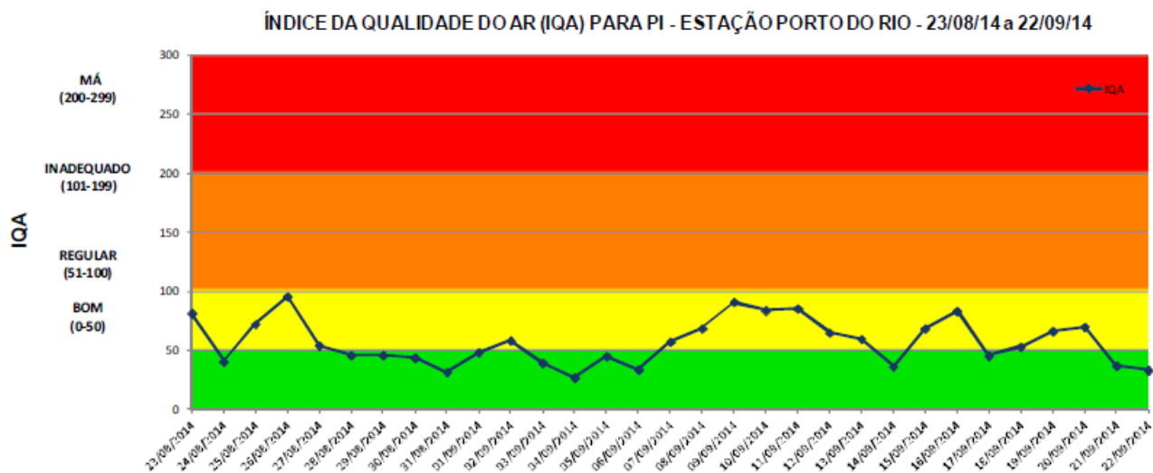
Figura: Variação temporal dos Índices de Qualidade do Ar para Partículas Inaláveis no período de 23/08/14 a 22/09/14 (Fonte: JCTM). Pontos de Medição: Inca.
