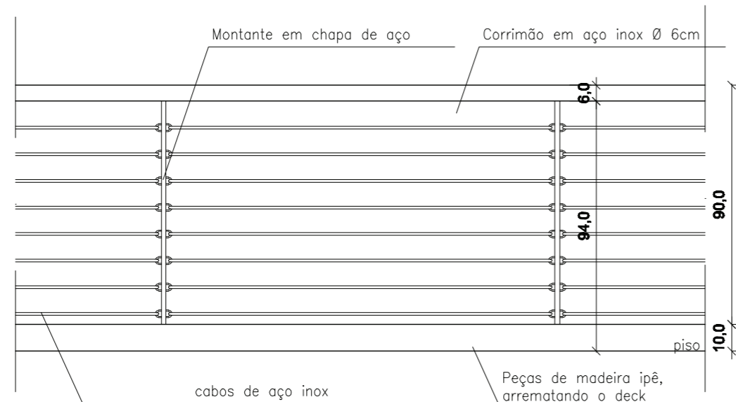
01 VISTA ESCALA 1/20
